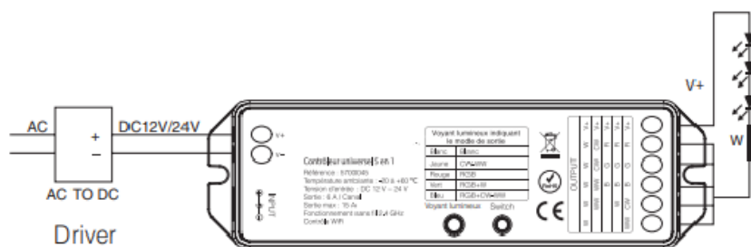
Connexion du contrôleur au ruban LED blanc
