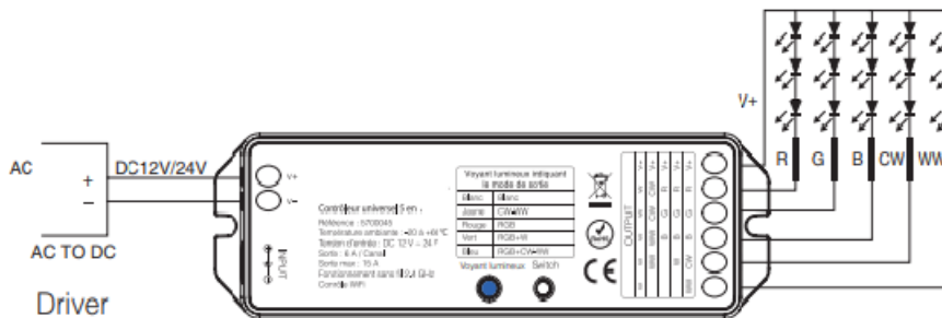
Connexion du contrôleur au ruban LED RGB+CW-WW
