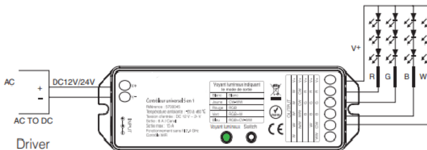
Connexion du contrôleur au ruban LED RGB+W
