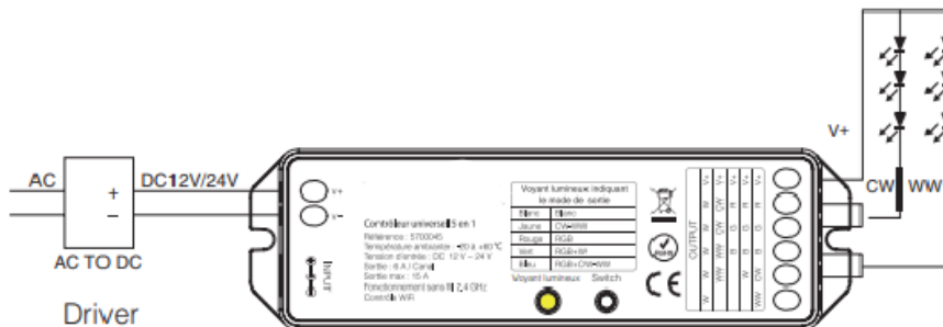
Connexion du contrôleur au ruban LED CW-WW
