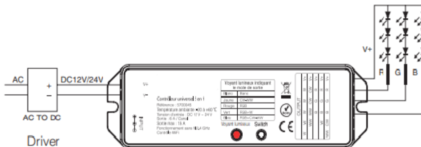
Connexion du contrôleur au ruban LED RGB
