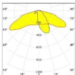
Optique routier
